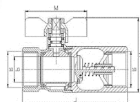
VÁLVULA ESFERA C/ RETENÇÃO LATÃO F/F 3/4 GENEBRE
